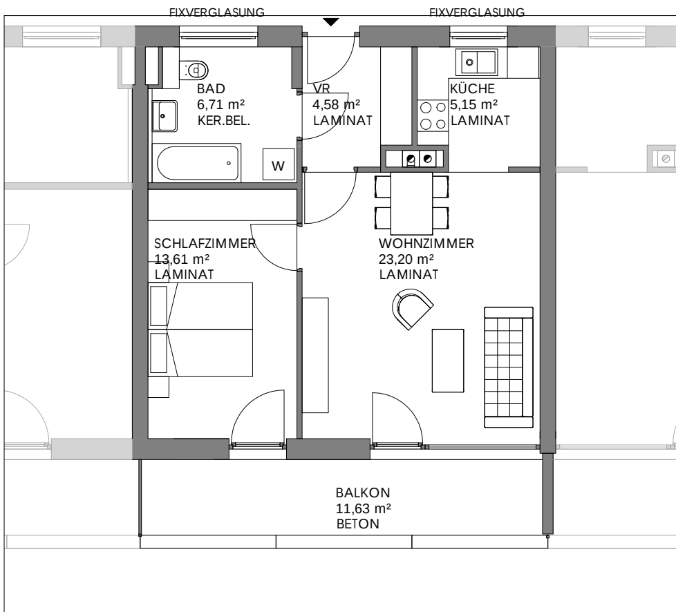
GRUNDRISS WOHNUNG M 1:100
