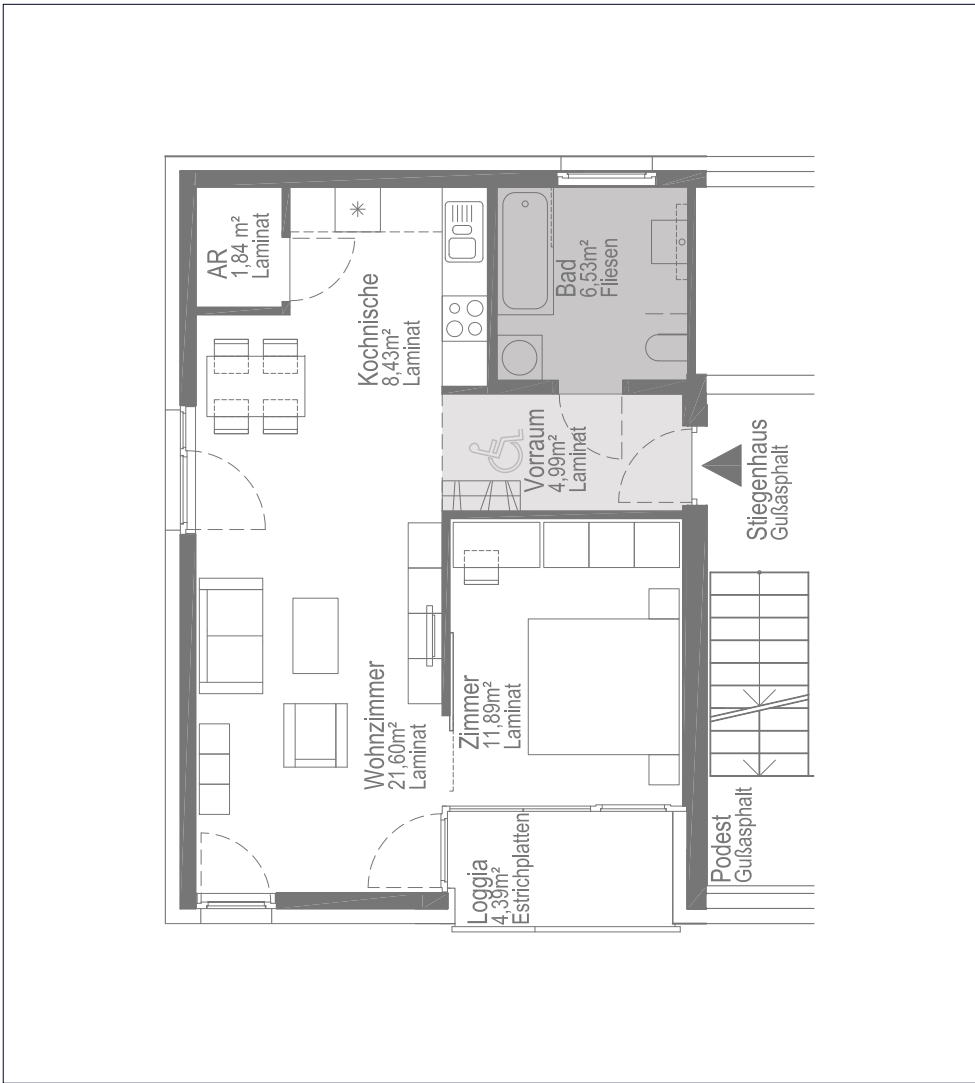
GRUNDRISS WOHNUNG
