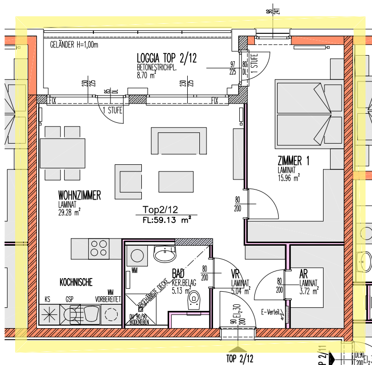
1. OBERGESCHOSS TOP 2/12
