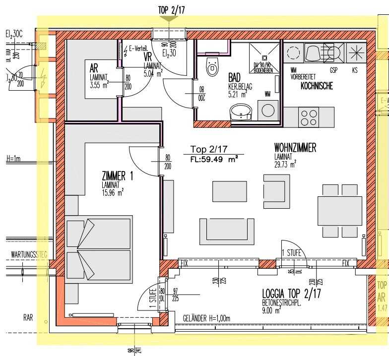
2. OBERGESCHOSS TOP 2/17
