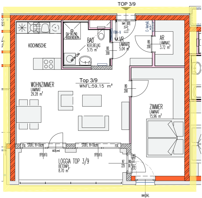
1. OBERGESCHOSS TOP 3/9
